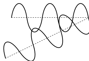
Interferencia destructiva
