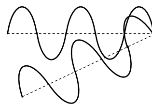
Interferencia constructiva
